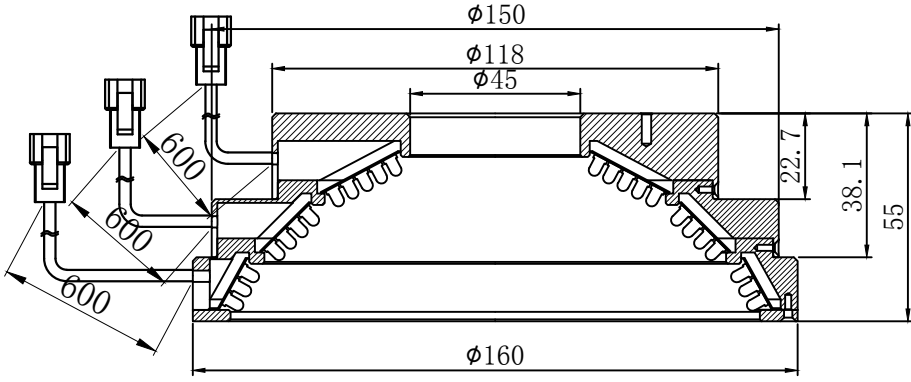
剖面 A-A
